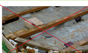
Zkontrolujte, zda jsou mezi nosníky expanzní spoje 10 mm
