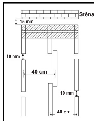
Příklad odsazené instalace
